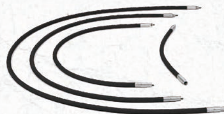
EJES FLEXIBLES SUPERFLEX Longitud de 1 a 4 m Longitud (pies): 13 | Peso (kg): 7,3 Código Superflex 10 - 967859501 Código Superflex 20 - 967859503 Código Superflex 30 - 967859504 Código Superflex 40 - 967859505
